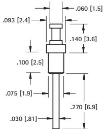
Feed-Thru
