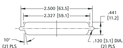
BNC
