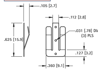
DWG. 2 MATERIAL: .010 (.25) Brass
