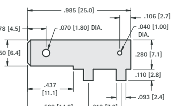
.250 (6.4) TAB
