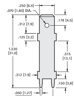
.250 (6.4) TAB
